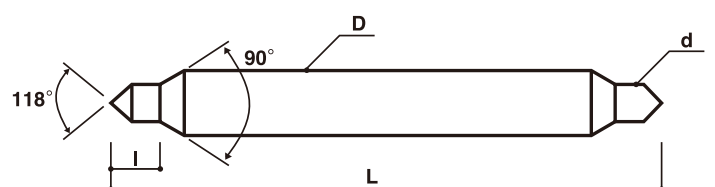
材質 SKH59
